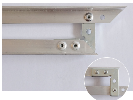
Indstøbningsrammer til nedstøbning i brønden.
