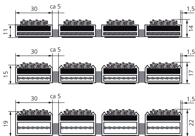
Entrance ALU med nålefilt i tre forskellige højde.
