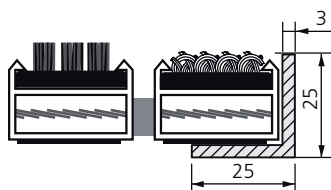
Nålefilt (R) og kassettebørste (CB) i indstøbningsramme
