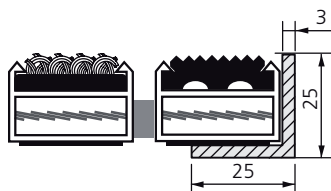
Nålefilt (R) og gummi (G) i indstøbningsramme
