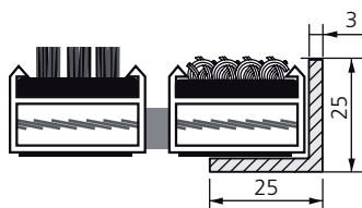
Nålfilt (R) och kassettborst (CB) i ingjutningsram
