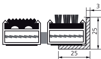
Gummi (G) och kassettborst (CB) i ingjutningsram
