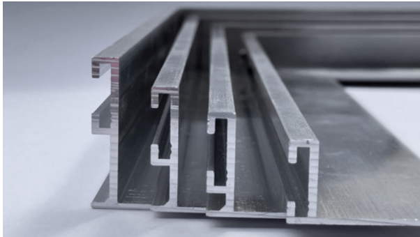
Ingjutningsram aluminium (natur)
