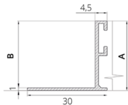
Ingjutningsram aluminium (natur)
